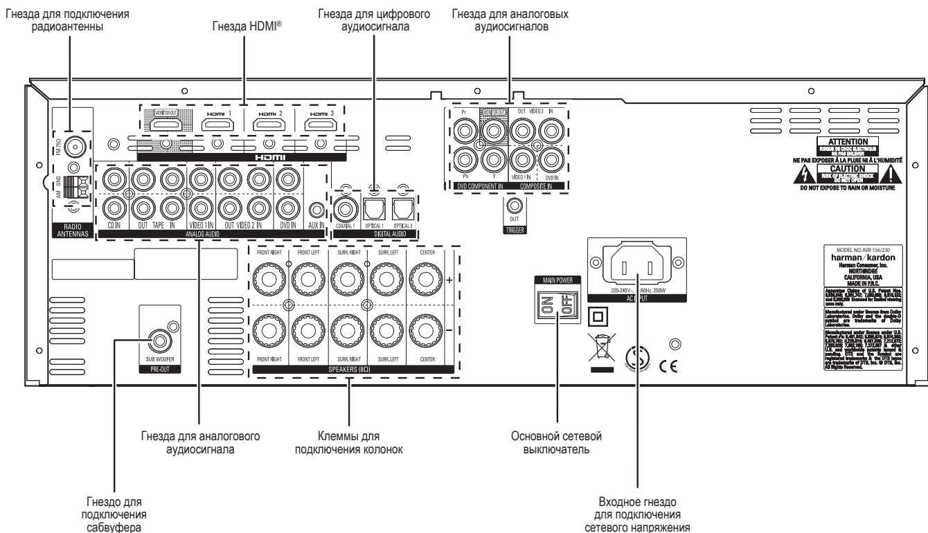
AVR 156 Схема подключений на задней панели
